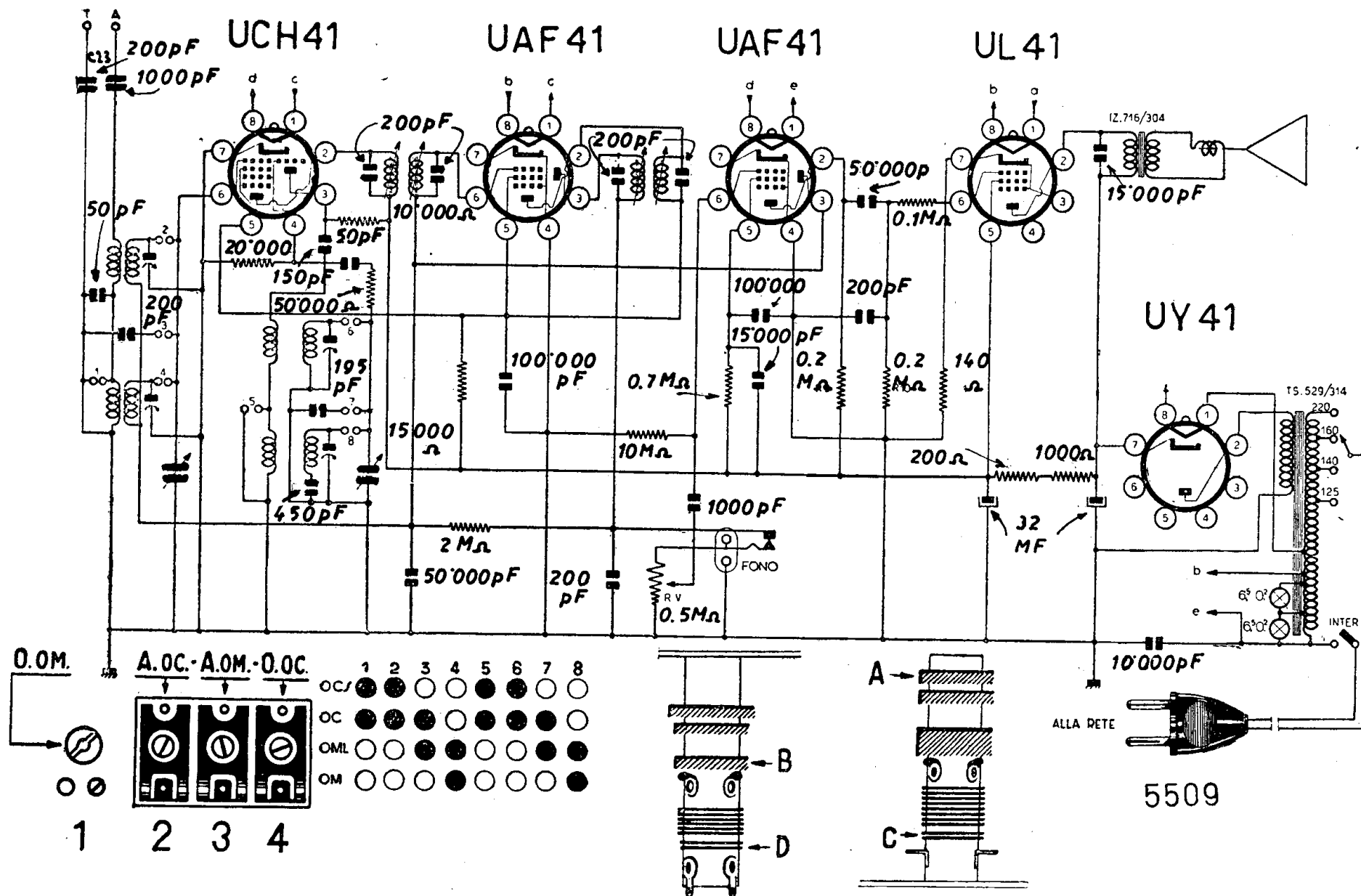
PHONOLA RADIO - Mod. 5509 - Medie e corte divise. MF a 470 kc. Placca finale 174 V, schermo 158; placca convertitrice 158 V, schermo 70, placca triodo 100 V; placca e schermo amplif. MF 70 V. Funicella come 5519.
